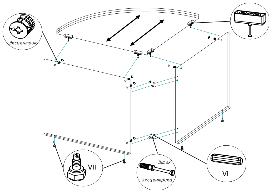
Рис. 2 Угловой элемент правый
