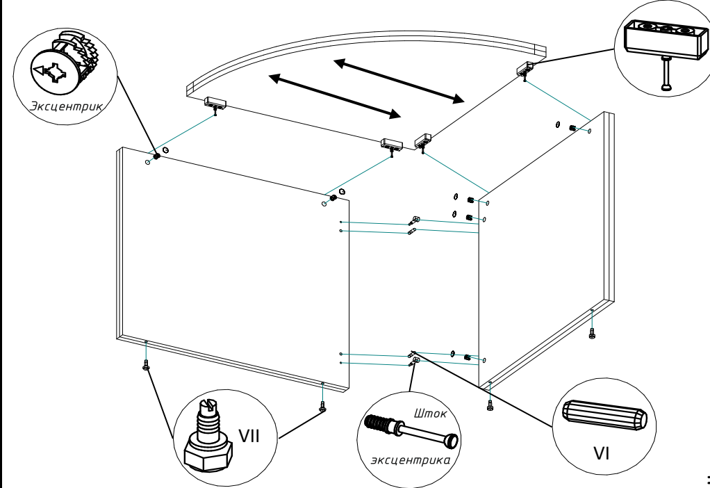
Рис. 2 Угловой элемент левый
